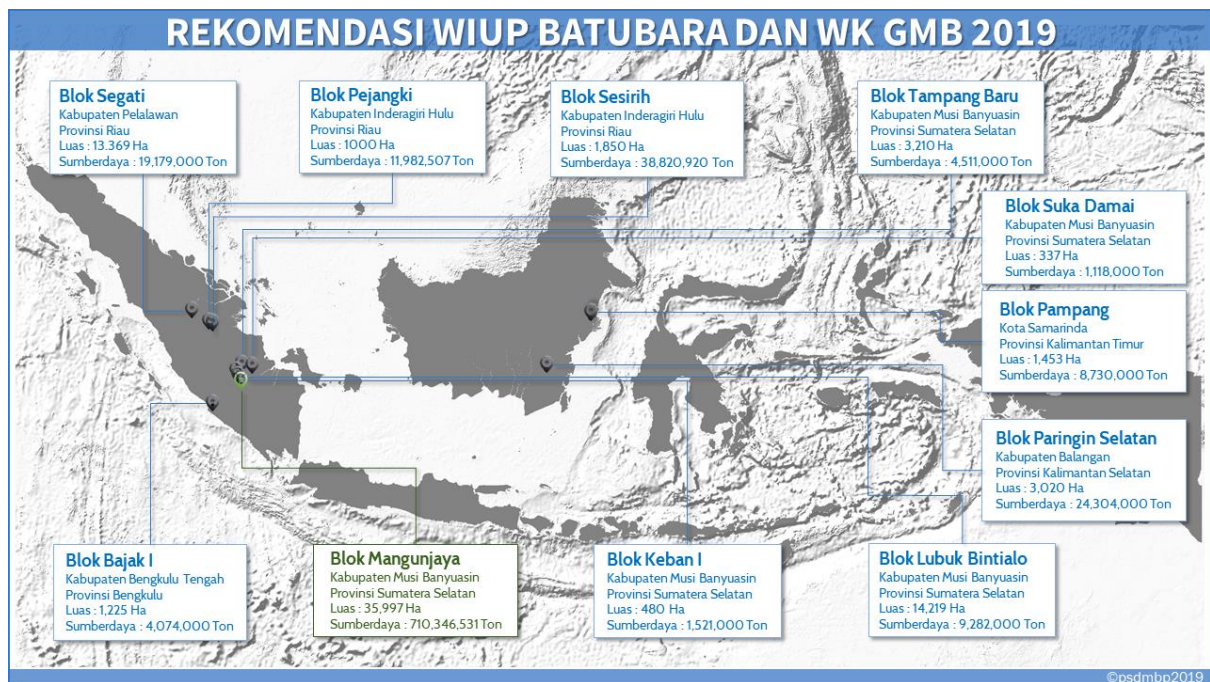
Gambar 3.15Peta usulan WIUP batubara dan WK GMB tahun 2019
