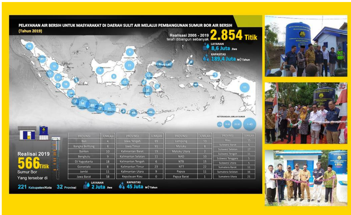
Gambar 3.4 Capaian Layanan Sumur Bor sampai Tahun 2019
