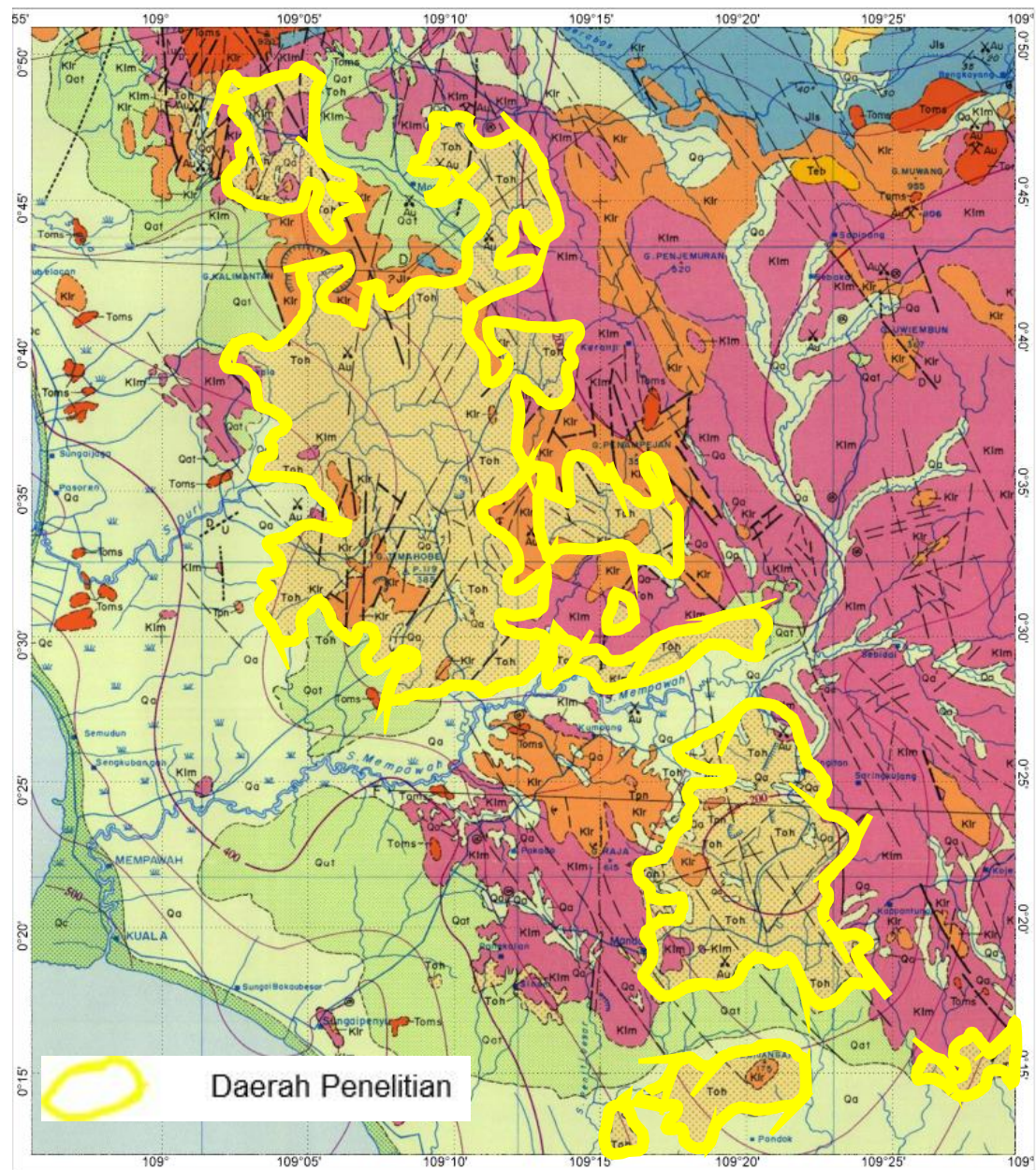
Gambar 3.10 Daerah Penelitian WK Singkawang.
