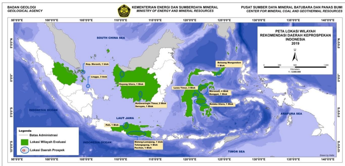
Gambar 3.16. Peta lokasi rekomendasi WIUP Mineral tahun 2019
