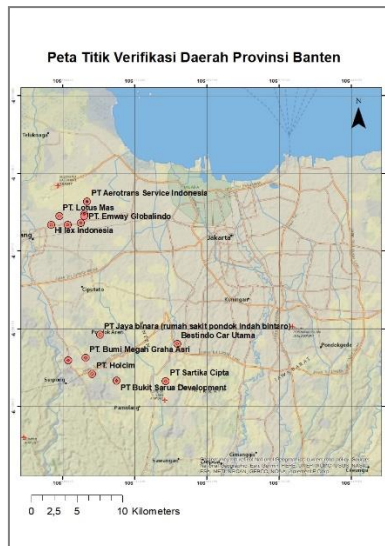
Gambar 3.7 Lokasi pemohon rekomendasi teknis pemanfaatan air tanah Provinsi Banten yang diverifikasi tahun 2019.
