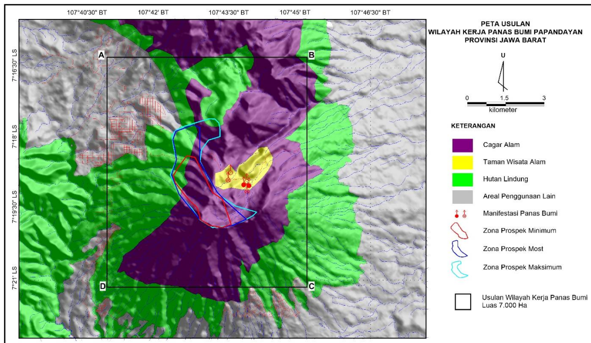
Gambar 3.13 Peta rekomendasi WK daerah panas bumi Papandayan.
