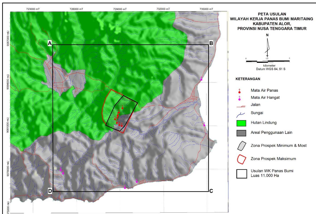
Gambar 3.14 Peta rekomendasi WK daerah panas bumi Maritaing.
