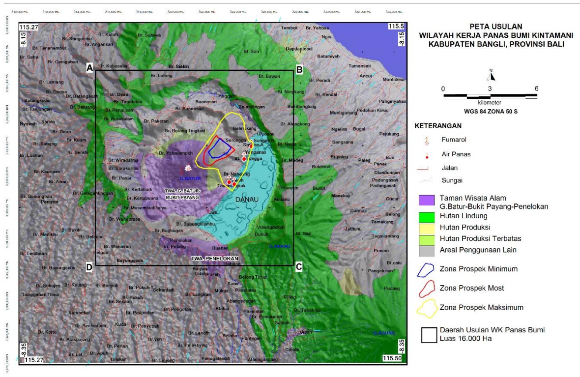
Gambar 3. 12 Peta rekomendasi WK panas bumi Kintamani.
