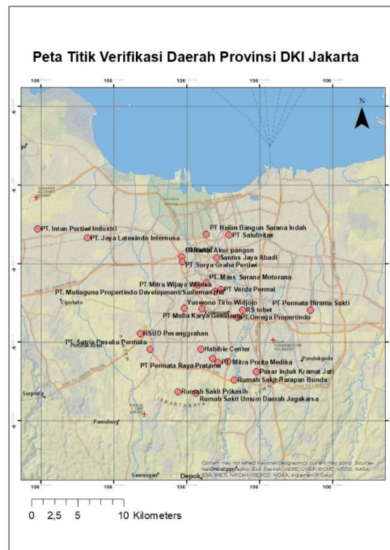
Gambar 3.6 Lokasi pemohon rekomendasi teknis pemanfaatan air tanah Provinsi DKI Jakarta yang diverifikasi tahun 2019.
