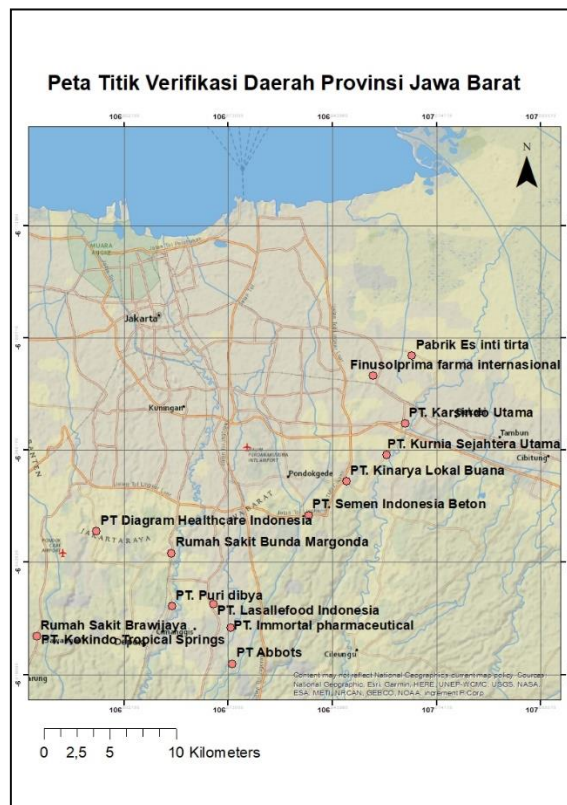
Gambar 3.8 Lokasi pemohon rekomendasi teknis pemanfaatan air tanah Provinsi Jawa Barat yang diverifikasi tahun 2019.
