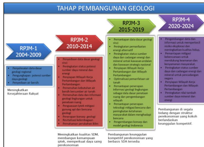
Gambar 3.1 Tahap Pembangunan Geologi Jangka Panjang 2004-2024
